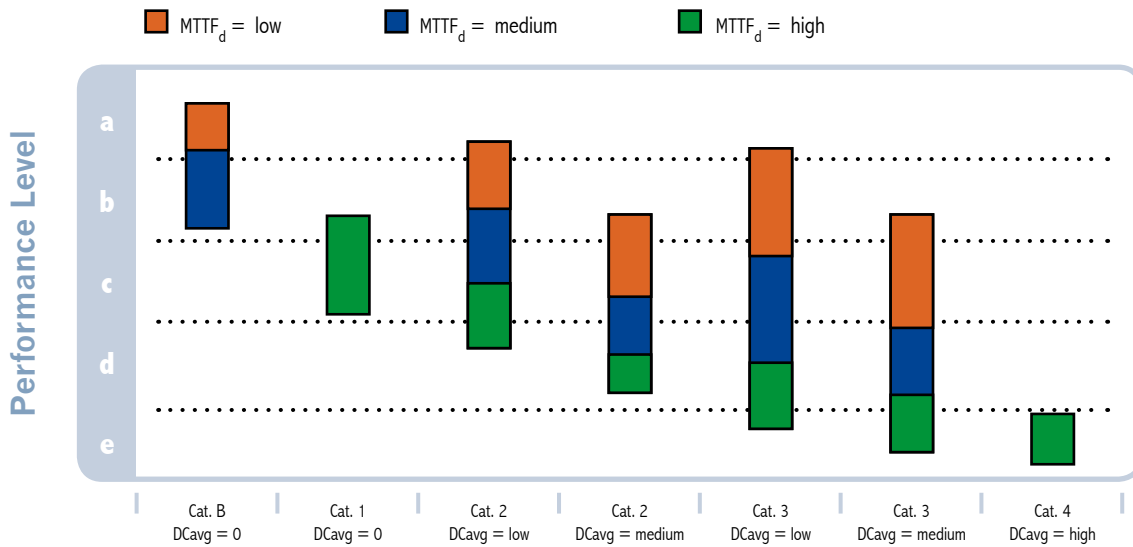
Fig. 5 of ISO 13849-1
